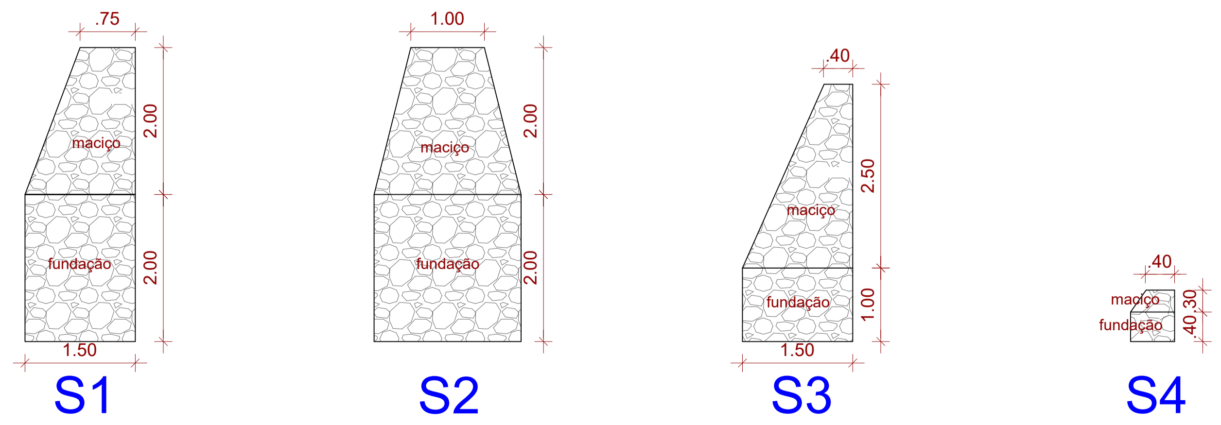
SEÇÕES DOS MUROS DE ARRIMO - SÍTIO FIGUEIRAS ESCALA _____ 1/50
